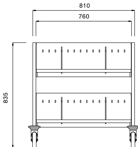
Front aanzicht
