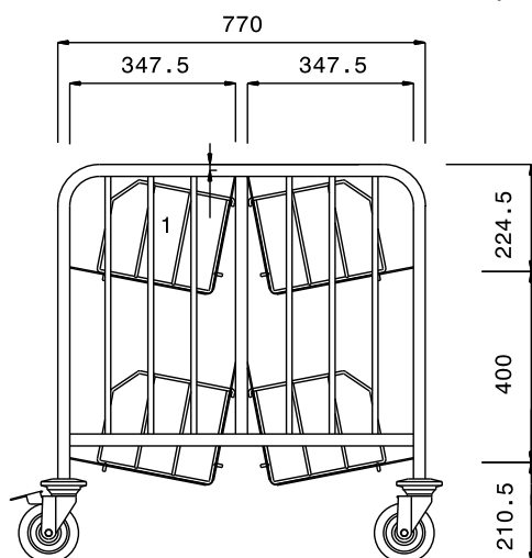
Zij aanzicht
